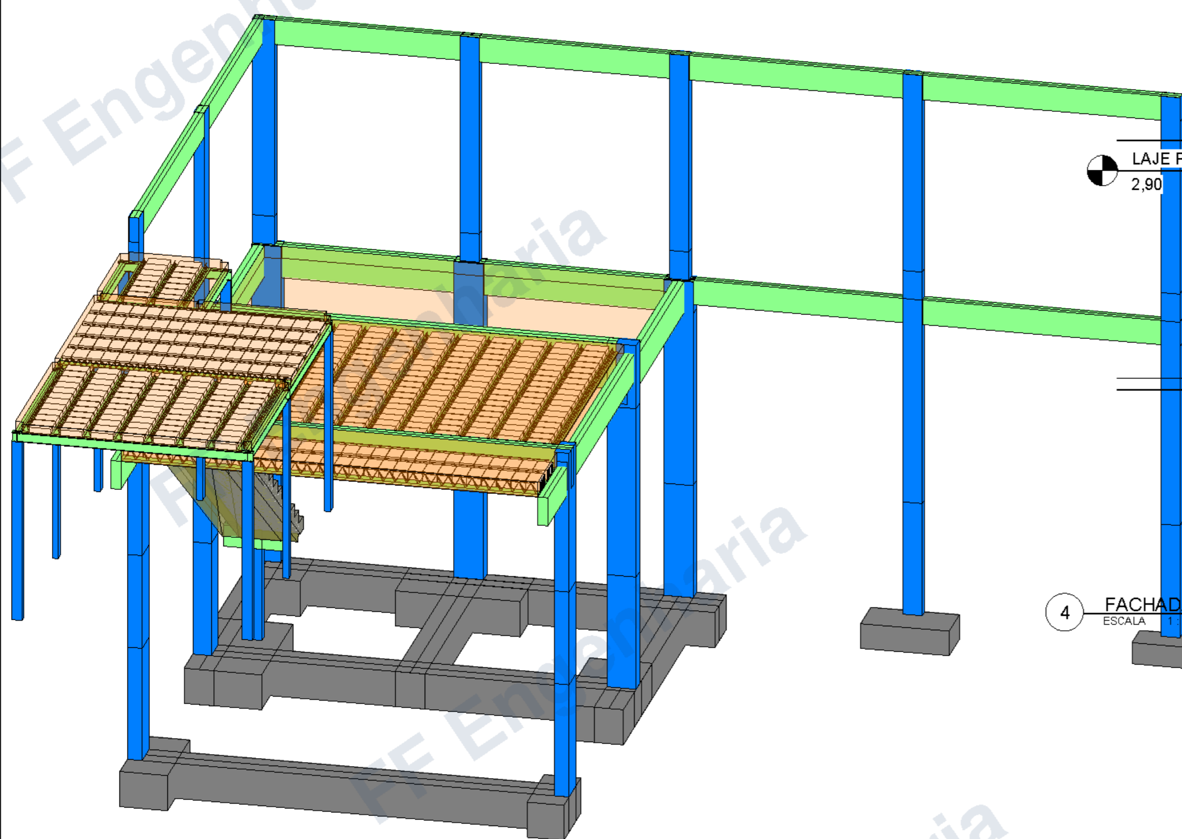
2 Estrutura piscina 2 ESCALA
